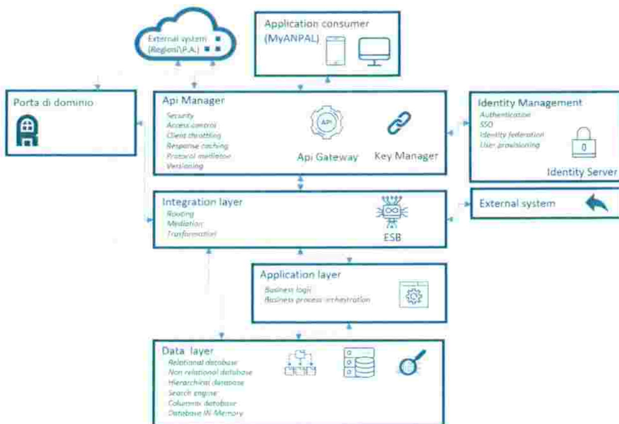
Figura 2 - Architettura logica del Sistema per la gestione dei flussi di dati amministrativi e della condizionalità
