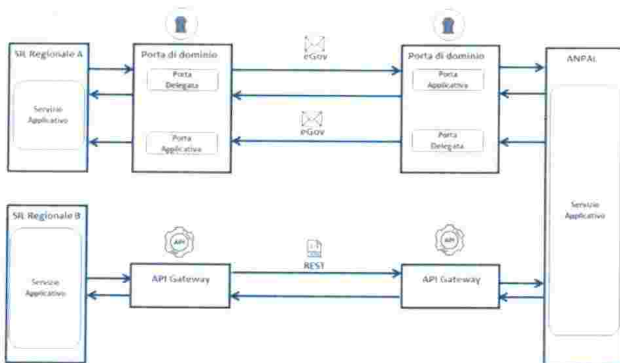
Figura 3 - Flussi di cooperazione applicativa
